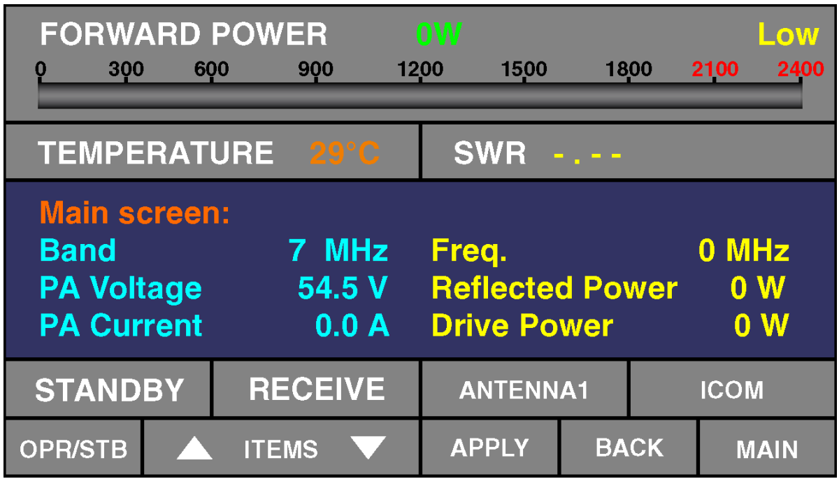
5-1. Меню «MAIN SCREEN» - выбор параметров усилителя на главной странице меню
